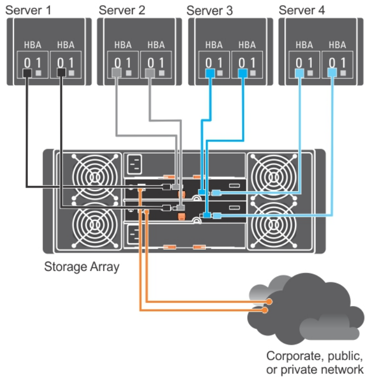
Figure 2. Quatre hôtes connectés à deux contrôleurs
