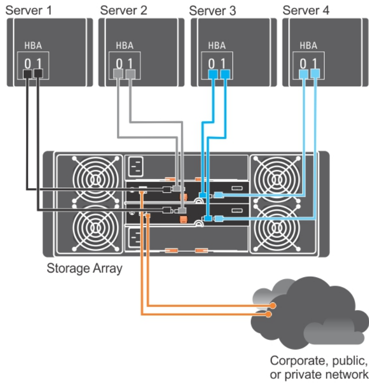
Figure 3. Quatre hôtes connectés à deux contrôleurs
