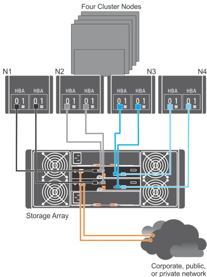
Figure 6. Quatre nœuds de clusters connectés à deux contrôleurs
