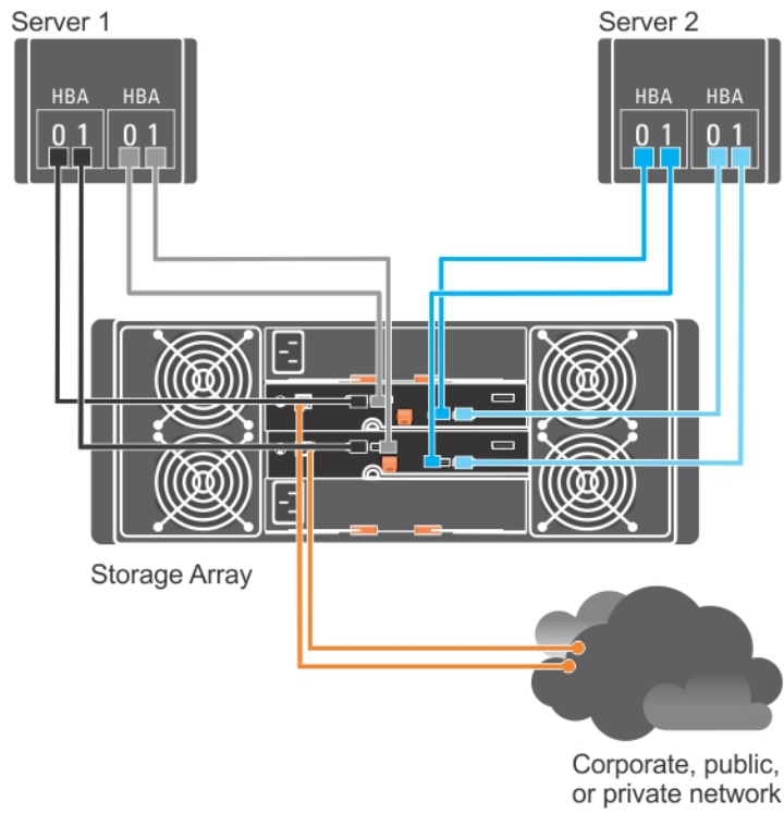
Figure 1. Deux hôtes connectés à deux contrôleurs
