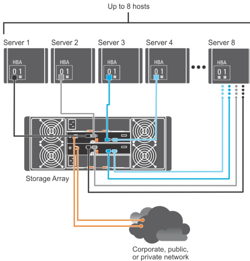
Figure 4. Huit hôtes connectés à deux contrôleurs
