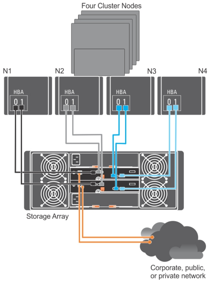
Figure 5. Quatre nœuds de clusters connectés à deux contrôleurs
